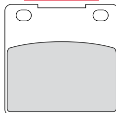
FDB338 53x53x9mm
