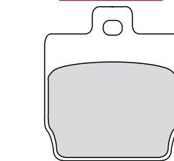
FDB2062 45.7x52.6x6.4mm
