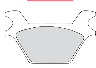
FDB2001 104x62x11.2mm
