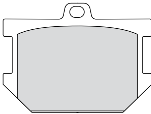
FDB177 62x45x11mm
