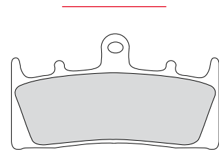
FDB873 90x52x8mm
