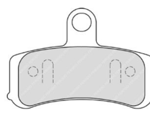
FDB2250 89x62x8mm
