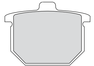
FDB182 69x49x9.5mm
