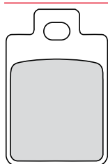
FDB2037 31.6x49x7mm
