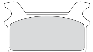
FDB485 104x62x12mm
