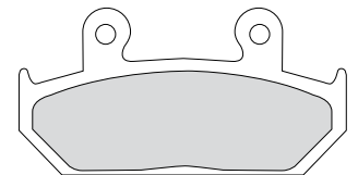
FDB663 88x46x9.8mm
