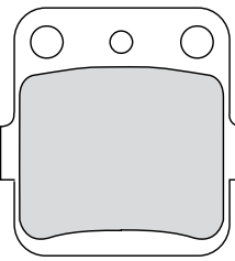
FDB381 46x45x7.3mm
