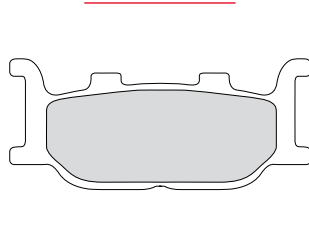
FDB2003 94x41x10mm
