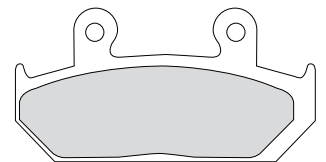
FDB452 88x46x8.3mm
