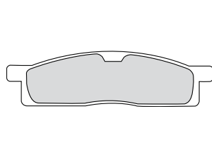
FDB2015 83x22x7mm
