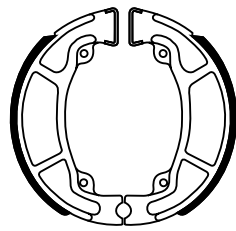
FSB963 125x25mm
