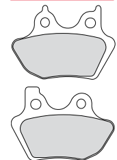
FDB2097 93.5x65x7.5mm
