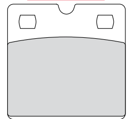
FDB204 60x59x9mm
