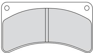
FDB2091 79.7x43.9x10.3mm
