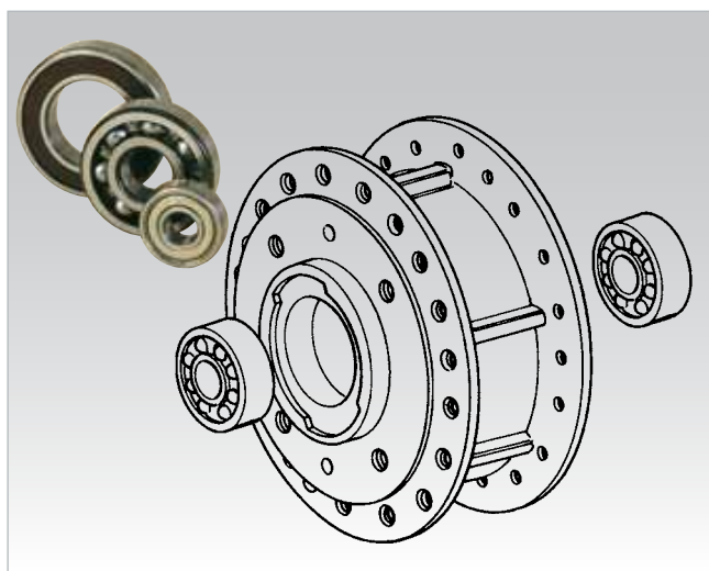
FRONT HUB • VOORNAAF • MOYEU AVANT
