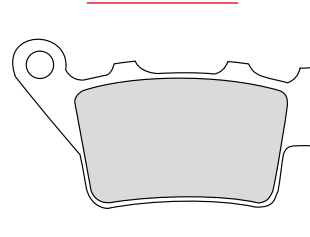
FDB2005 77x43x9mm
