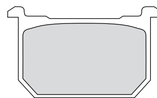
FDB298 68x41x9.5mm
