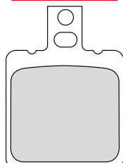
FDB207 40x57x7mm
