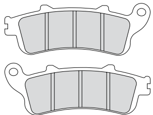
FDB2098 115.1x41x8.3mm
