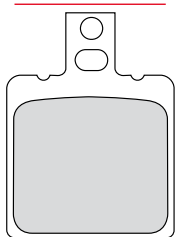
FDB705 40x57x8mm
