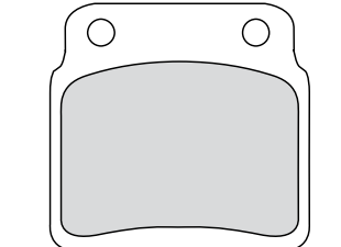
FDB2016 47x45x7.3mm
