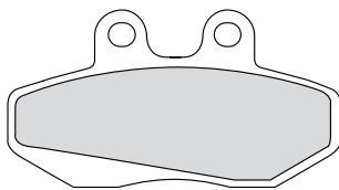
FDB706 76x46x7mm
